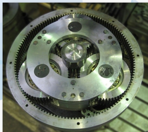
Планетарная передача редуктора углеразмольной мельницы
